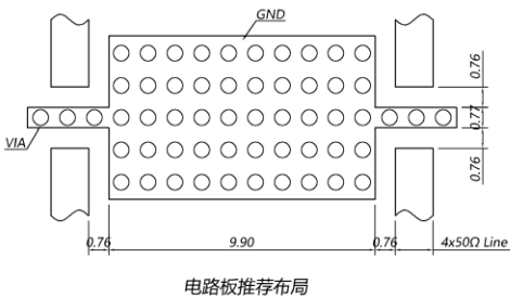
电路板推荐布局
